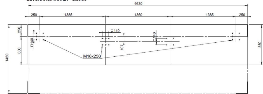
ZÁKLADOVÝ PAS / CONTINUOUS FOOTING / FUNDAMENTSTREIFEN VAR A KUBATURA BETONU / CONCRETE CUBATURE / BETONRAUMINHALT - 2.36m 3
